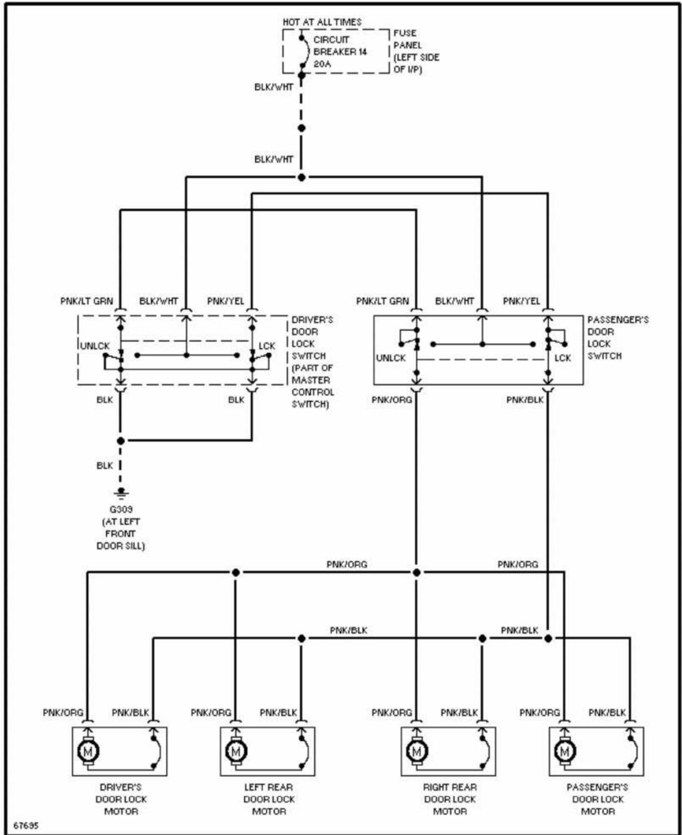
Fig. 8: Door Lock Circuit 1989 Ford Taurus LX
