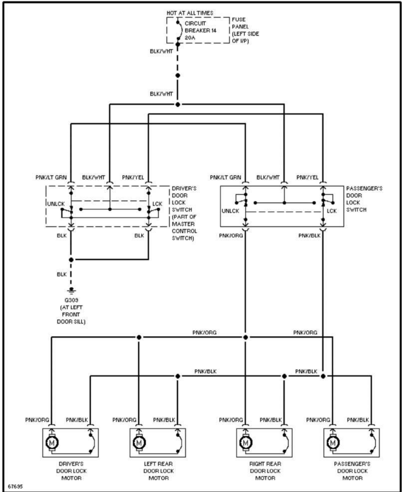
Fig. 8: Door Lock Circuit 1991 Ford Taurus LX
